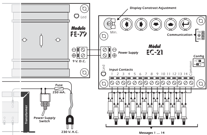
Fig. 1. General Wiring Map.
