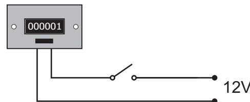
Activación mediante pulsador, final de carrera, etc.
