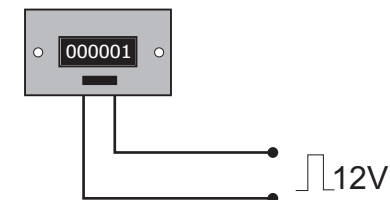
Activación mediante impulsos de 12V.
