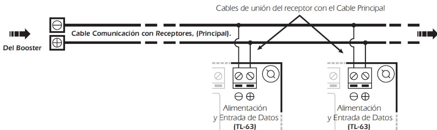
Fig. 1. Conexión entre el Recetor y el Booster.
