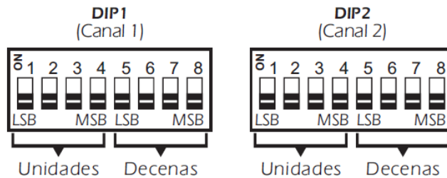
Fig. 5. Configuración de los switches según el número introducido.
