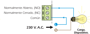
Fig. 3. Filtro anti-Fluctuación relé.
