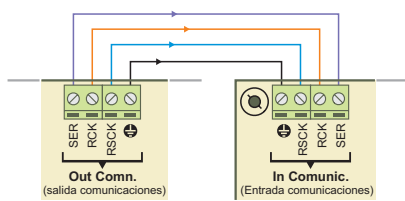
Fig. 1. Conexión Entre receptor y placa esclava.
