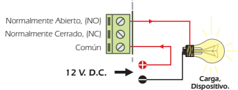
Fig. 2. Ejemplos de Conexión de la Carga.
