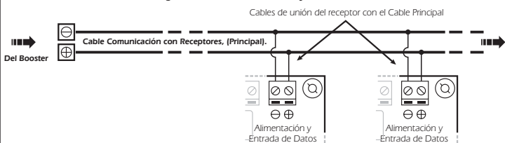
Fig. 1. Conexión entre el Receptor y el Booster.
