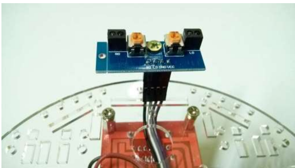
Figure 9 – 2 : Brancher le connecteur au capteur. Attention à la polarité.
