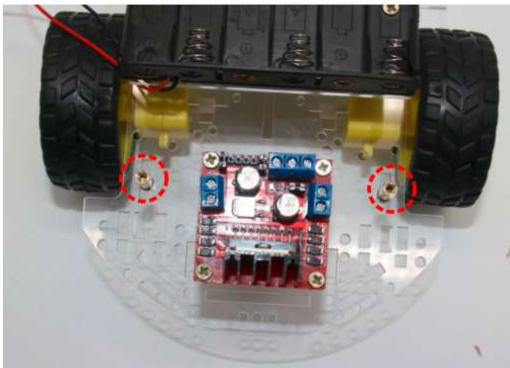
Figure 6- 2 : Installation des deux séparateurs à l'aide de vis M3 x 10mm .
