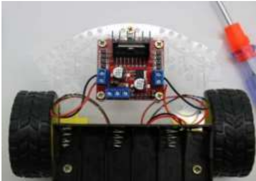
Figure 7- 3 : Connecter les câbles du moteur gauche à la partie gauche du module de contrôle des moteurs (bornes A1 et A2) et ceux du moteur de droite à la partie droite (bornes B1 et B2)
