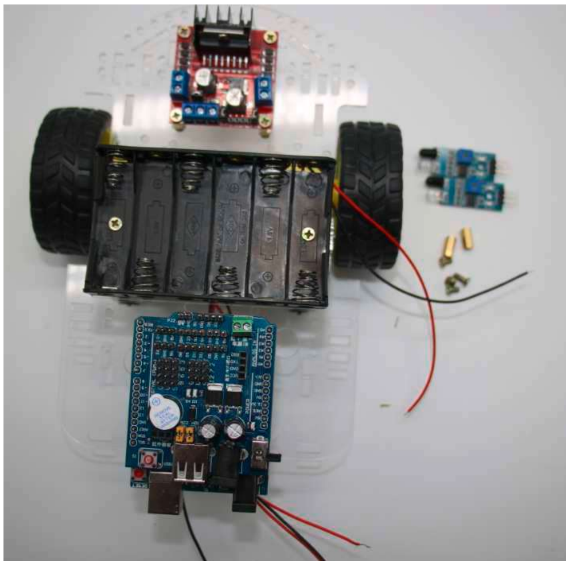
Figure 6 - 1 : Pièces nécessaires
