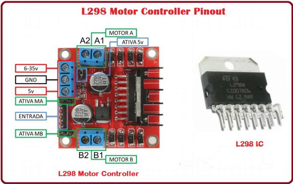
Figura 6 - 3 Conectar los cables del motor izquierdo a la parte izquierda del módulo controlador de motores (bornes A1 y A2) y los del motor derecho a la parte derecha (bornes B1 y B2)
