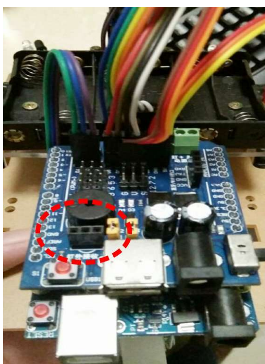
Figura 8 - 3 Situación del zócalo donde hay que enchufar el receptor de infrarrojos.
