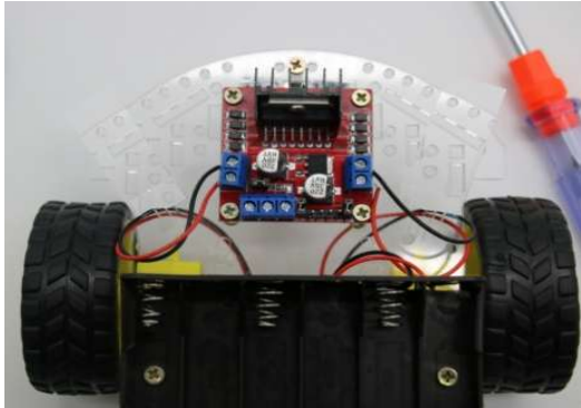
Figura 6 - 3 Conectar los cables del motor izquierdo a la parte izquierda del módulo controlador de motores (bornes A1 y A2) y los del motor derecho a la parte derecha (bornes B1 y B2)
