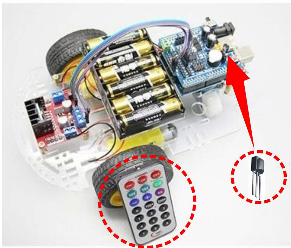
Figura 8 – 1 : Mando a distancia (izquierda) y receptor de infrarrojos (derecha)
