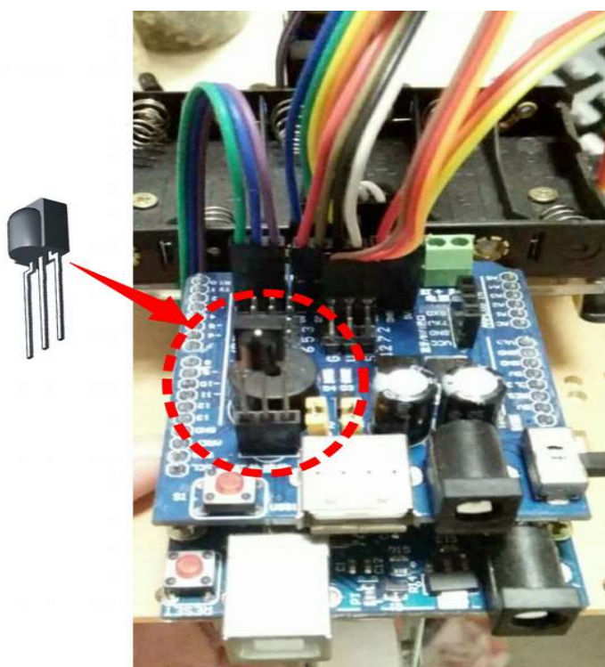
Figura 8 - 4 Vista de la posición correcta del receptor
