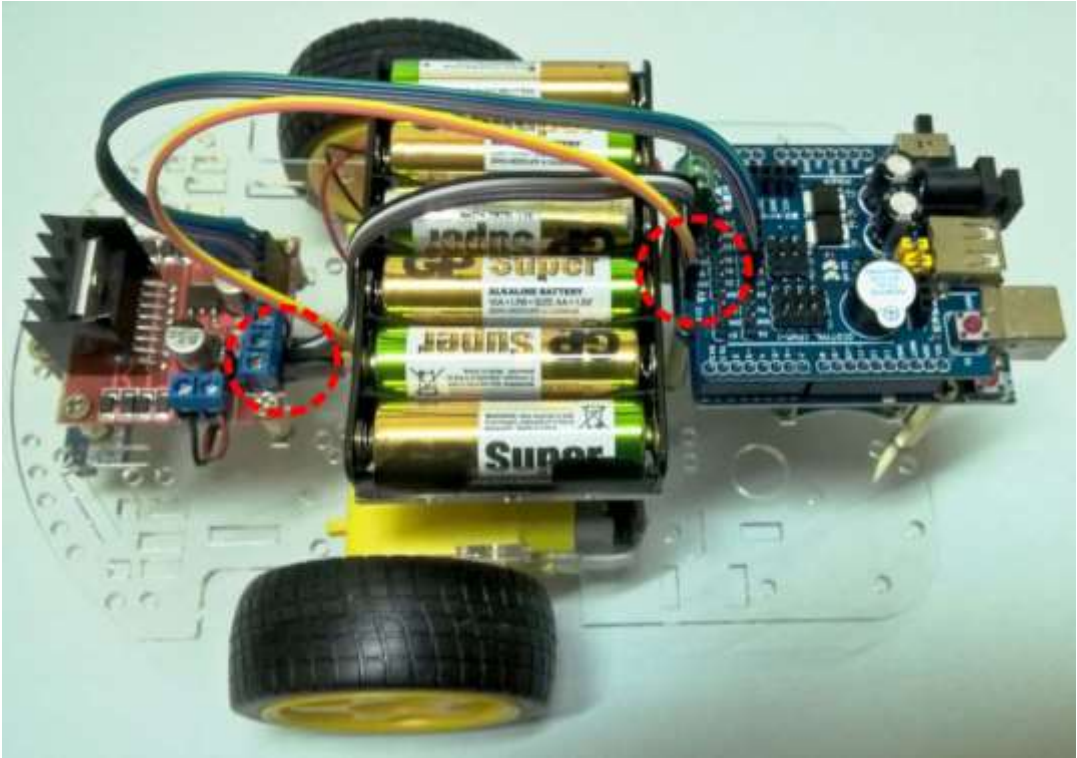
Figure 7 –9 : Vue du robot complètement terminé, où il est possible d’apprécier la connexion de l’alimentation du module de contrôle des moteurs. Les couleurs des câbles peuvent varier selon le modèle photographié.
