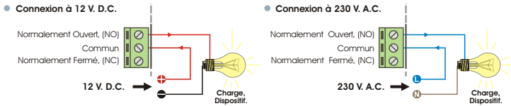
Fig. 1. Exemples de Connexion de la Charge.
